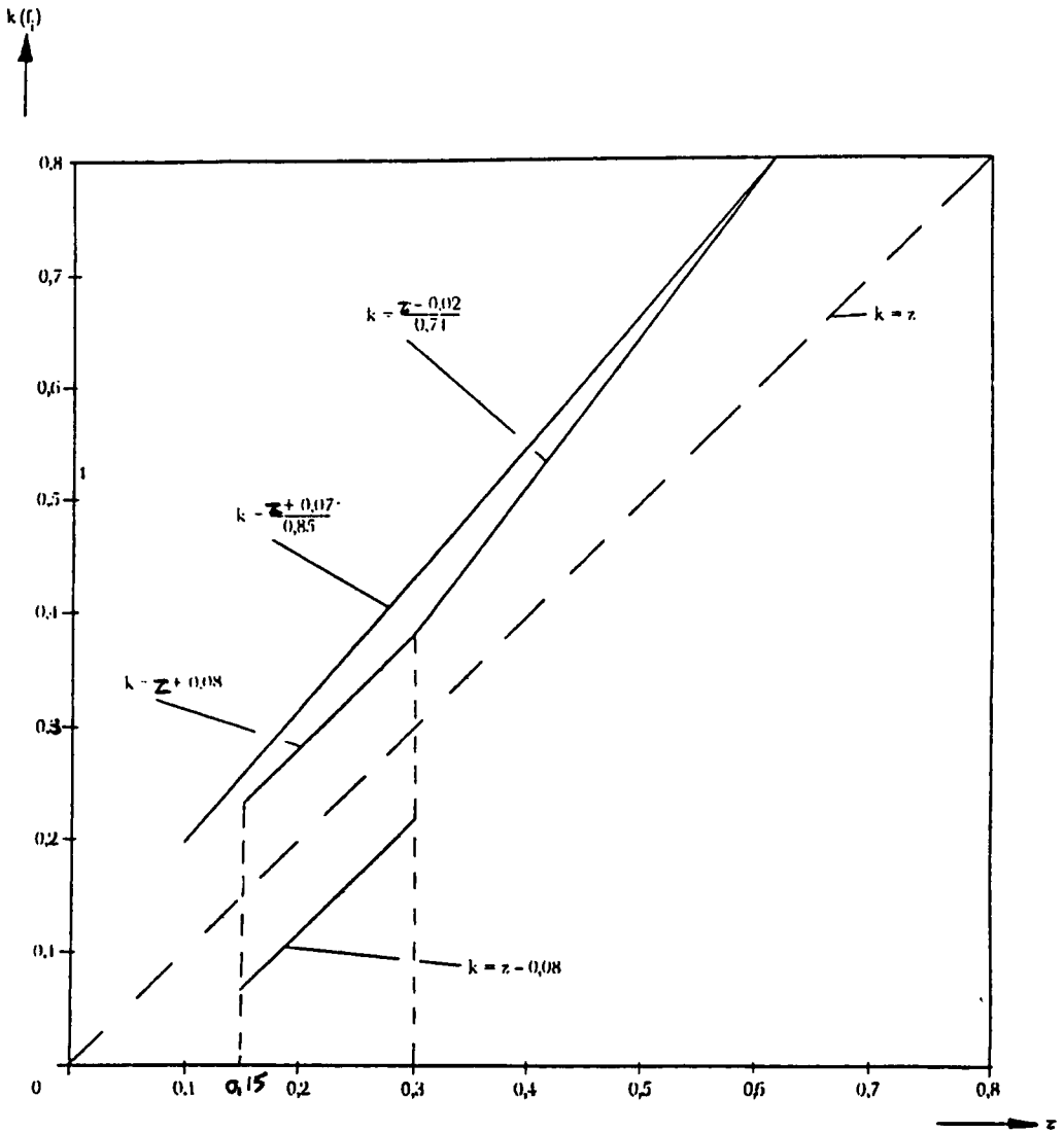
«Diagramme 1 B. VÉHICULES À MOTEUR AUTRES QUE CEUX DE LA CATÉGORIE M 1 «(Voir paragraphe 3.1.1)
