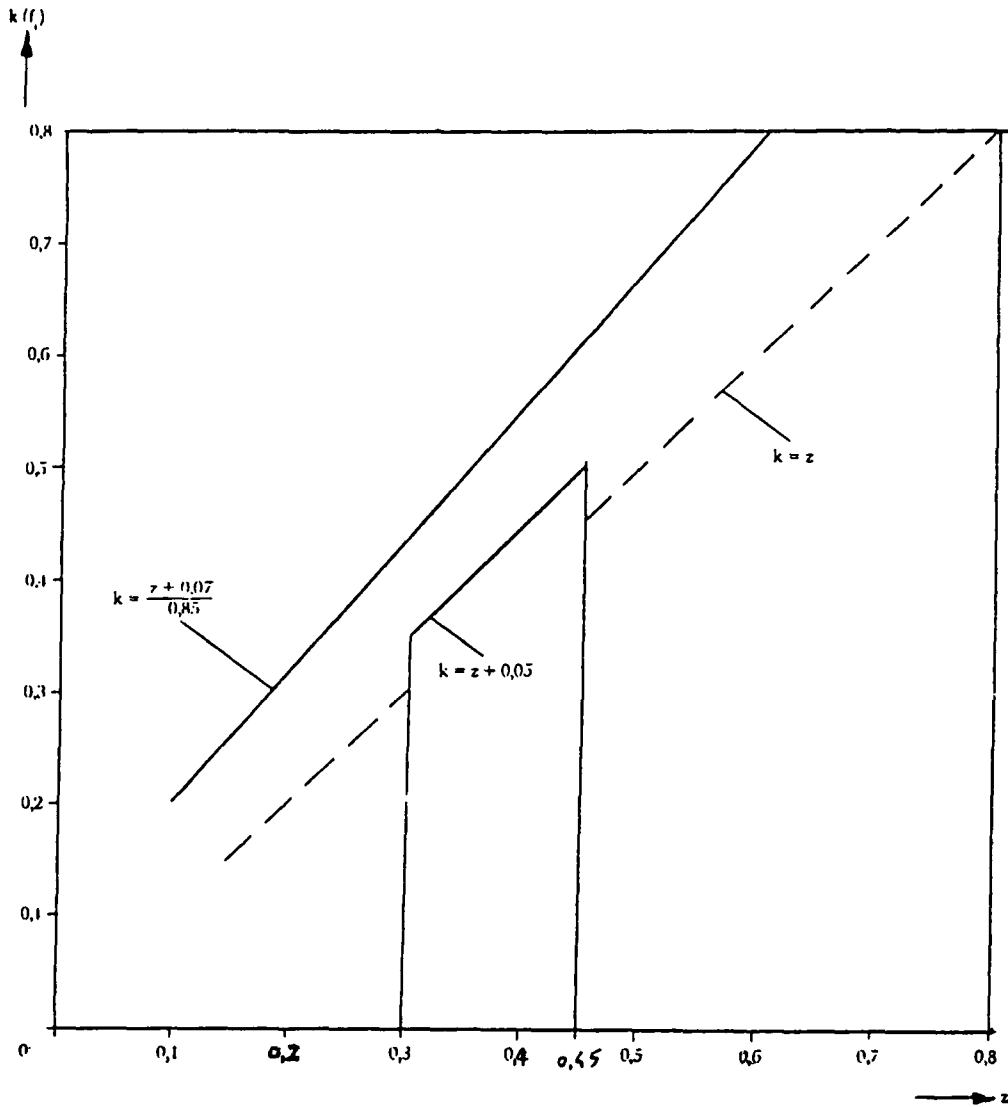
«Diagramme 1 A. VÉHICULES DE LA CATÉGORIE M 1 «(Voir paragraphe 3.1.1)
